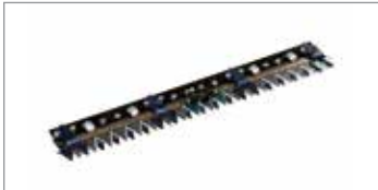
Lastrón completo central 1,15 m Dientes especiales Protecciones laterales Código 69229069A
